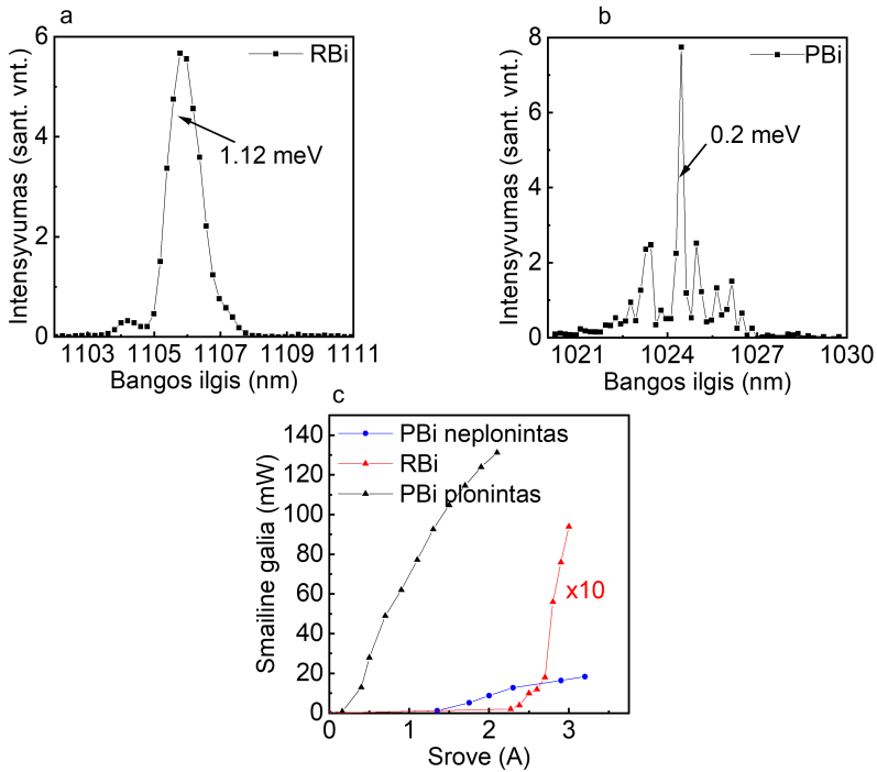
3.42 paveikslas: Lazerinių diodų lazeriavimo spektrai: a) prietaisui, veikiančiam standartinių stačiakampių kvantinių duobių pagrindu; b) prietaisui su parboliškai graduotais barjeriais (spektruose a) ir b) 1,12 meV ir 0,2 meV atitinka centrinės emisijos linijos FWHM); c) lazerinių diodų smailinės galios priklausomybė nuo įveikinimo srovės: stačiakampių kvantinių duobių lazeriui (raudona) ir lazeriams su parboliškai graduotais barjeriais – neplonintu padėklu (mėlyna) bei plonintu padėklu (juoda).
