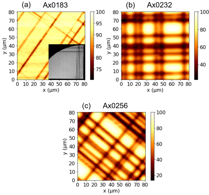
3.39 paveikslas: Ax0183, Ax0232 ir Ax0256 bandinių \mu PL žemėlapiai nuskenuoti iš 80 \times 80 \mu\text{m}^2 . Linijos išlygiuotos [0-1-1] ir [0-11] kryptimis. Įklijoje pateiktas RTPL žemėlapis, nuskenuotas iš stačiakampiu pažymėto ploto bandinyje Ax0183.
